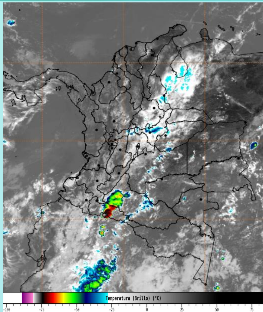
Imagen GOES 19 East Canal Infrarrojo, 9 de marzo de 2026 - Hora 11:50 HLC. Fuente: https://bart.ideam.gov.co GOES 19
