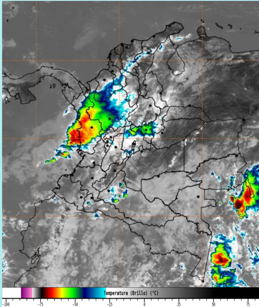
Imagen GOES 19 East Canal Infrarrojo, 8 de marzo de 2026 - Hora 11:50 HLC. Fuente: https://bart.ideam.gov.co GOES 19
