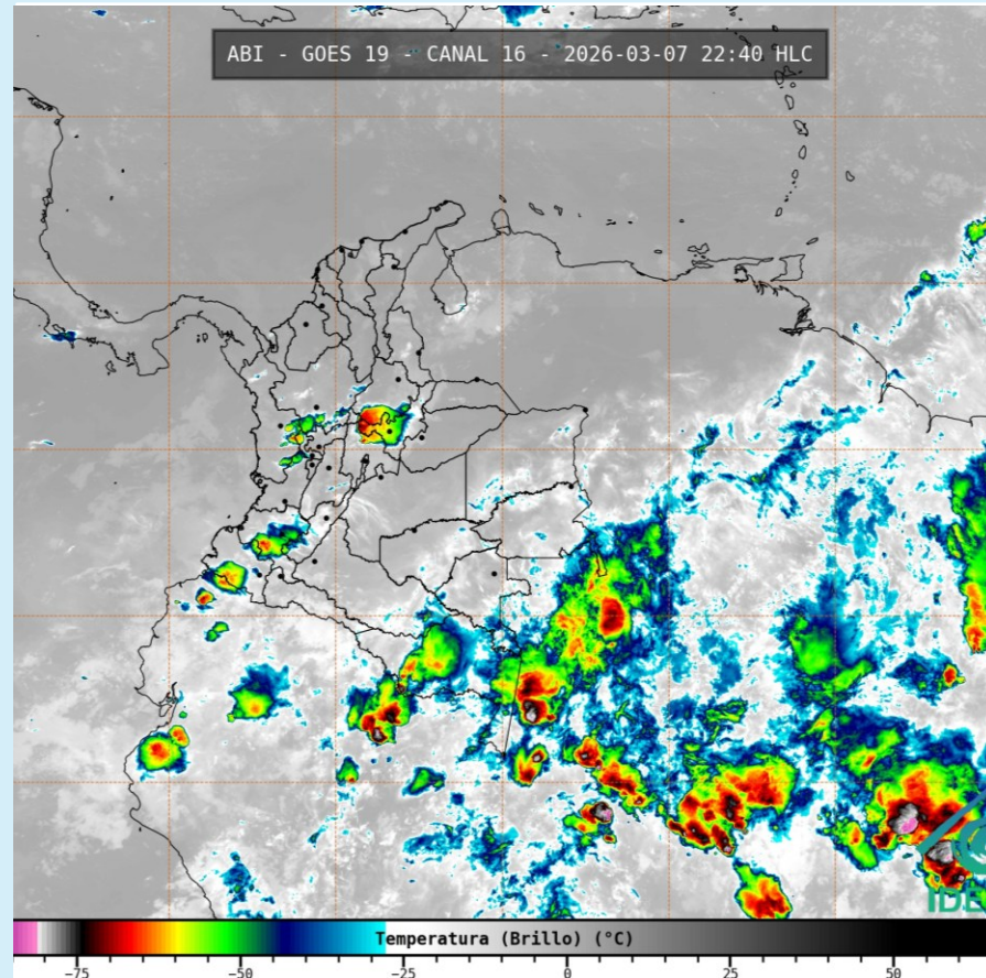
Imagen GOES 19 (East) Canal Infrarrojo 7 de marzo de 2026– Hora 22:40 HLC Fuente: IDEAM - GOES 19
