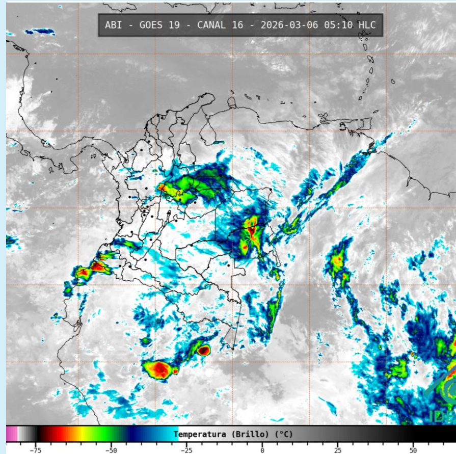
Imagen GOES 19 (East) Canal Infrarrojo 6 de marzo de 2026– Hora 05:10 HLC Fuente: IDEAM - GOES 19
