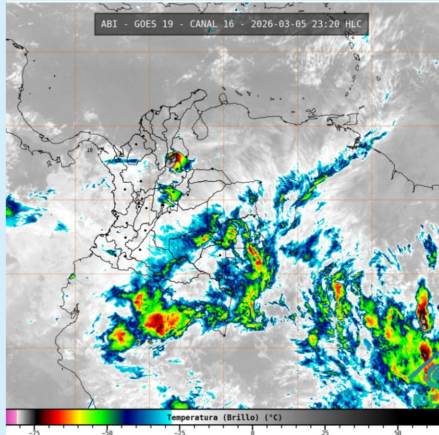
Imagen GOES 19 (East) Canal Infrarrojo 5 de marzo de 2026– Hora 23:20 HLC Fuente: IDEAM - GOES 19
