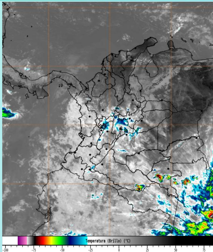
Imagen GOES 19 East Canal Infrarrojo, 5 de marzo de 2026 - Hora 12:00 HLC. Fuente: https://bart.ideam.gov.co GOES 19
