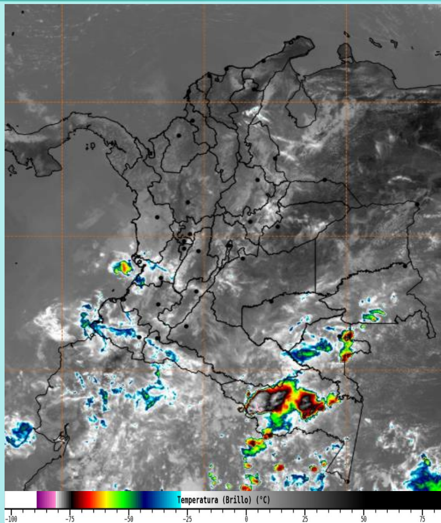
Imagen GOES 19 East Canal Infrarrojo, 2 de marzo de 2026 - Hora 12:10 HLC. Fuente: https://bart.ideam.gov.co GOES 19
