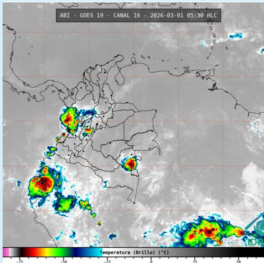
Imagen GOES 19 (East) Canal Infrarrojo 1 de marzo de 2026– Hora 05:30 HLC Fuente: IDEAM - GOES 19
