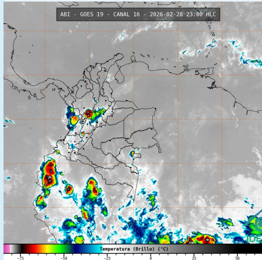
Imagen GOES 19 (East) Canal Infrarrojo 28 de febrero de 2026– Hora 23:00 HLC Fuente: IDEAM - GOES 19
