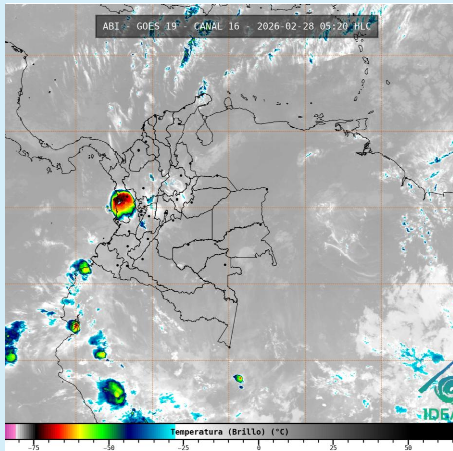
Imagen GOES 19 (East) Canal Infrarrojo 28 de febrero de 2026– Hora 05:20 HLC Fuente: IDEAM - GOES 19
