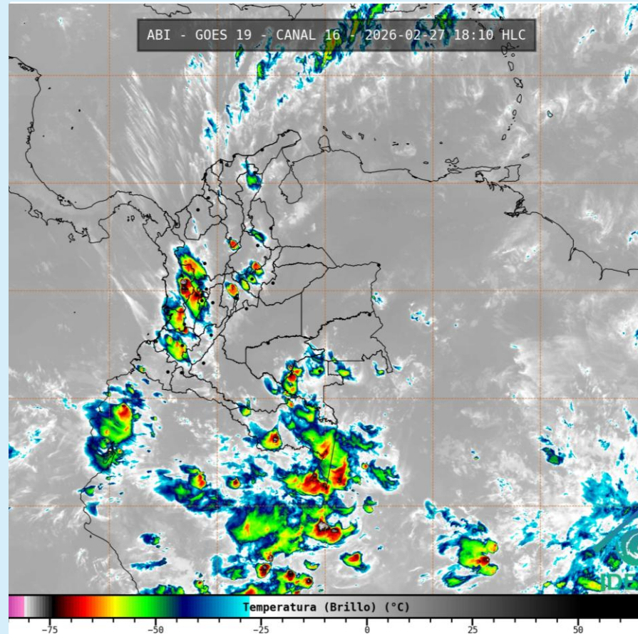
Imagen GOES 19 (East) Canal Infrarrojo 27 de febrero de 2026– Hora 18:10 HLC Fuente: IDEAM - GOES 19
