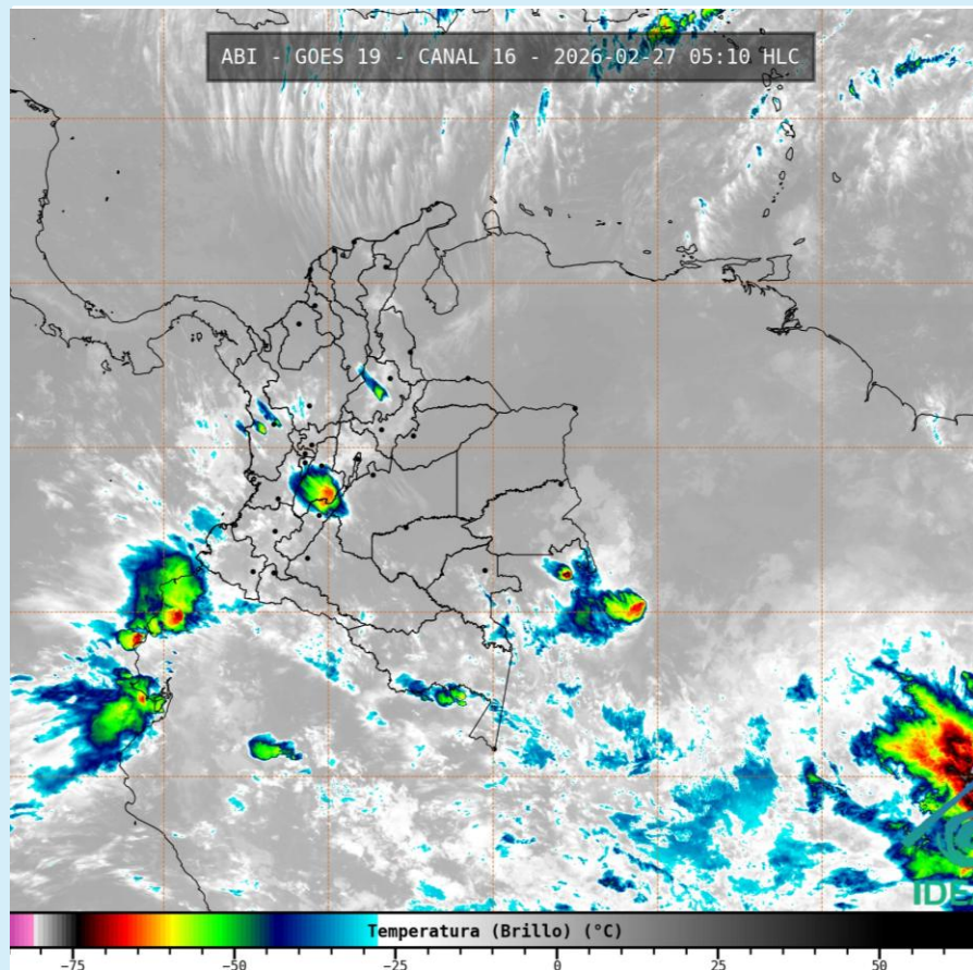
Imagen GOES 19 (East) Canal Infrarrojo 27 de febrero de 2026– Hora 05:10 HLC Fuente: IDEAM - GOES 19
