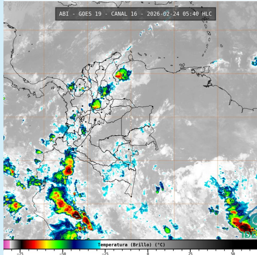
Imagen GOES 19 (East) Canal Infrarrojo 24 de febrero de 2026– Hora 05:40 HLC Fuente: IDEAM - GOES 19
