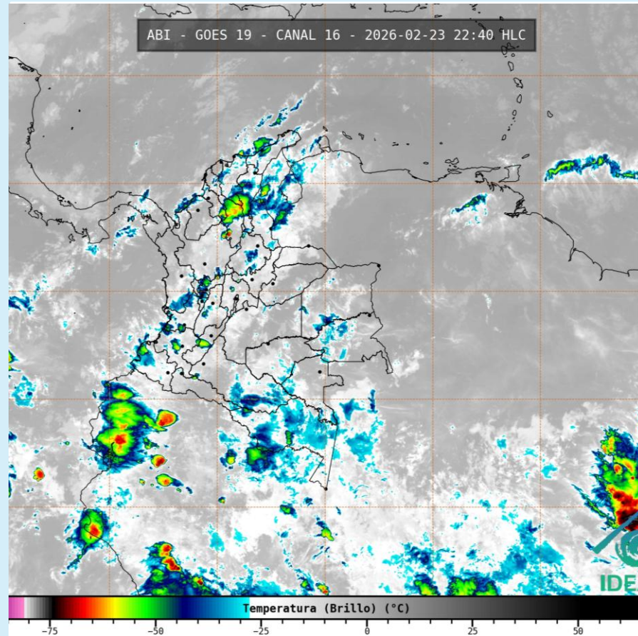
Imagen GOES 19 (East) Canal Infrarrojo 24 de febrero de 2026– Hora 22:40 HLC Fuente: IDEAM - GOES 19
