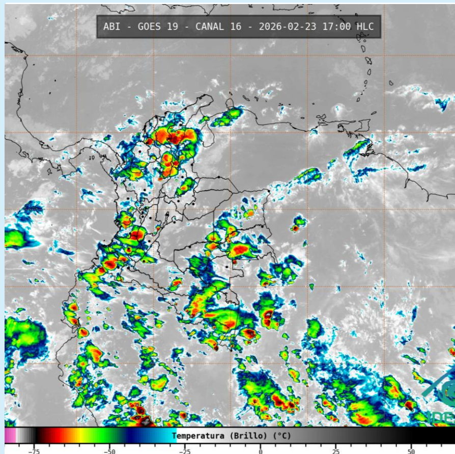
Imagen GOES 19 (East) Canal Infrarrojo 23 de febrero de 2026– Hora 05:40 HLC Fuente: IDEAM - GOES 19
