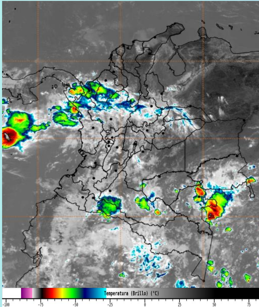
Imagen GOES 19 East Canal Infrarrojo, 22 de febrero de 2026 - Hora 12:00 HLC. Fuente: https://bart.ideam.gov.co GOES 19
