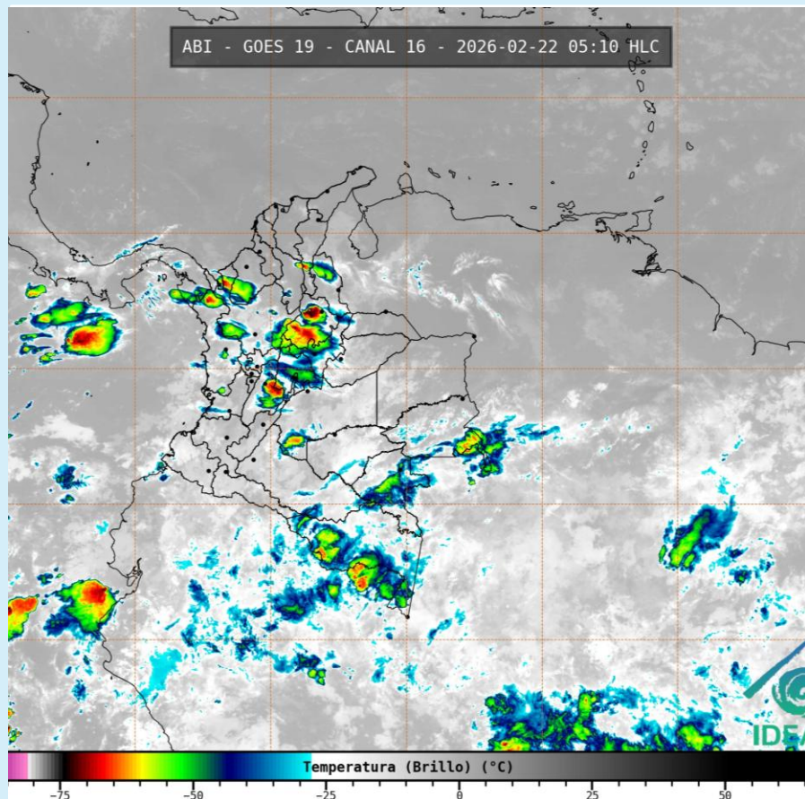
Imagen GOES 19 (East) Canal Infrarrojo 22 de febrero de 2026– Hora 05:10 HLC Fuente: IDEAM - GOES 19
