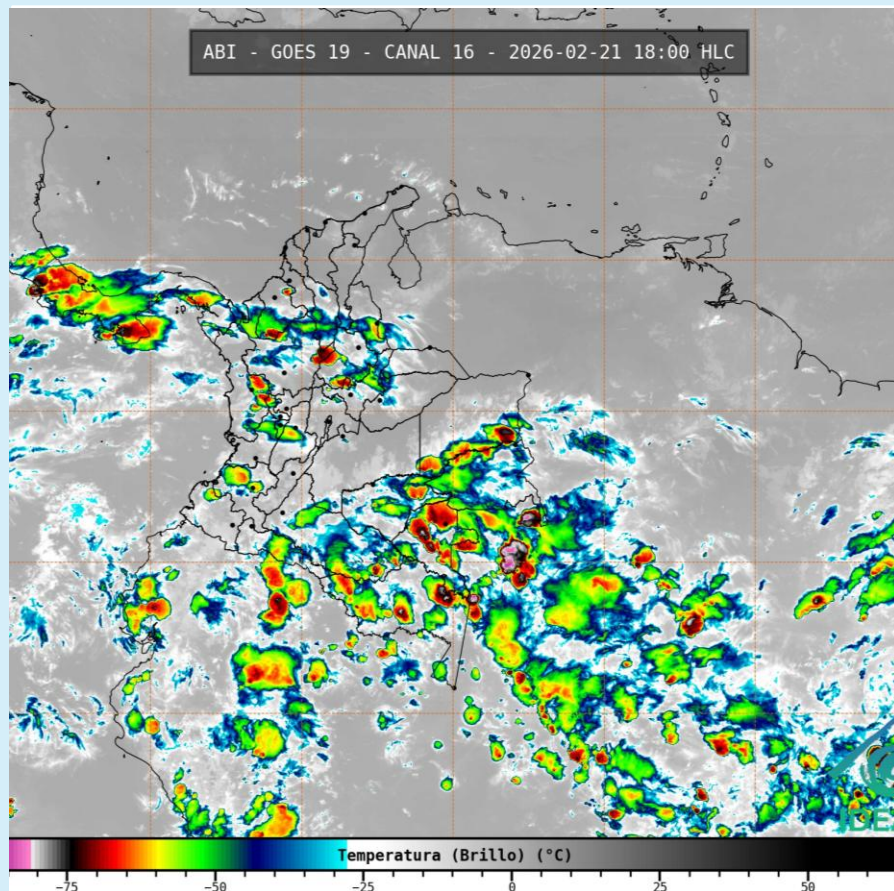
Imagen GOES 19 (East) Canal Infrarrojo 21 de febrero de 2026– Hora 18:00 HLC Fuente: IDEAM - GOES 19
