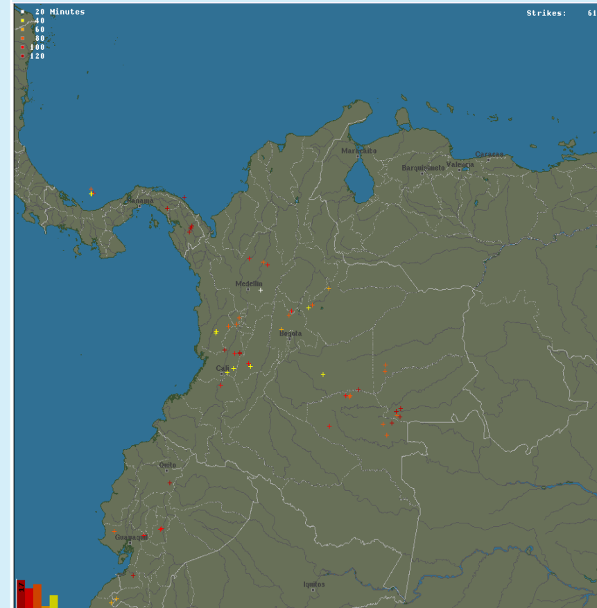
Descargas eléctricas (últimas horas) 19 de febrero de 2026 – Hora entre las 15:50 - 17:50 HLC Fuente: IDEAM - NOAA
