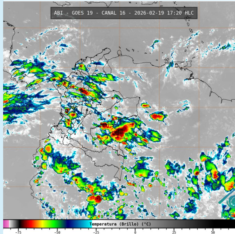
Imagen GOES 19 (East) Canal Infrarrojo 19 de febrero de 2026– Hora 17:20 HLC Fuente: IDEAM - GOES 19
