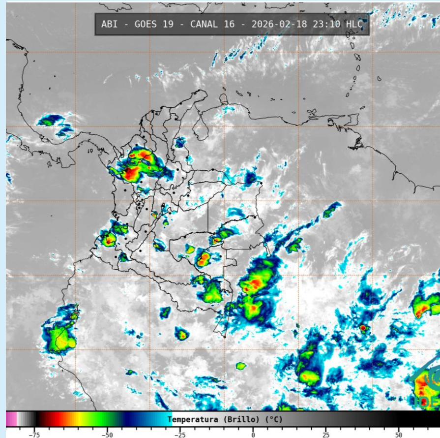
Imagen GOES 19 (East) Canal Infrarrojo 18 de febrero de 2026– Hora 23:10 HLC Fuente: IDEAM - GOES 19
