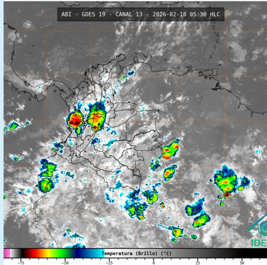
Imagen GOES 19 (East) Canal Infrarrojo 18 de febrero de 2026– Hora 05:30 HLC Fuente: IDEAM - GOES 19
