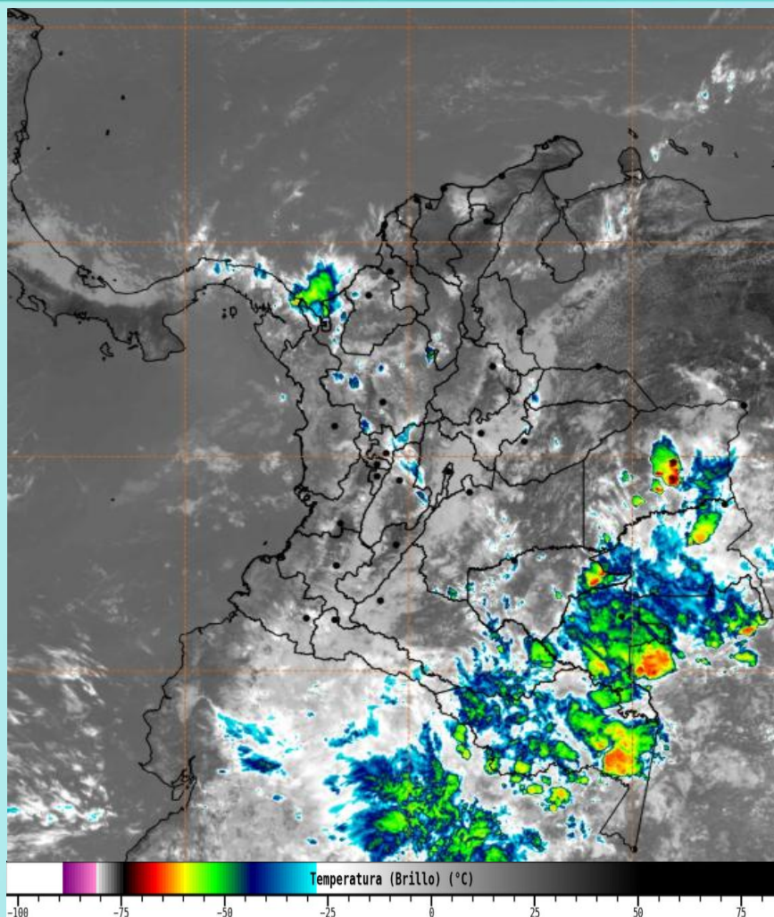
Imagen GOES 19 East Canal Infrarrojo, 17 de febrero de 2026 - Hora 12:10 HLC. Fuente: https://bart.ideam.gov.co GOES 19
