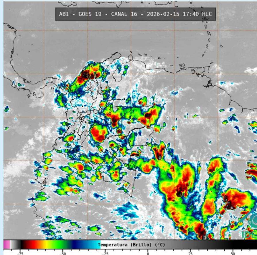
Imagen GOES 19 (East) Canal Infrarrojo 15 de febrero de 2026– Hora 17:40 HLC Fuente: IDEAM - GOES 19
