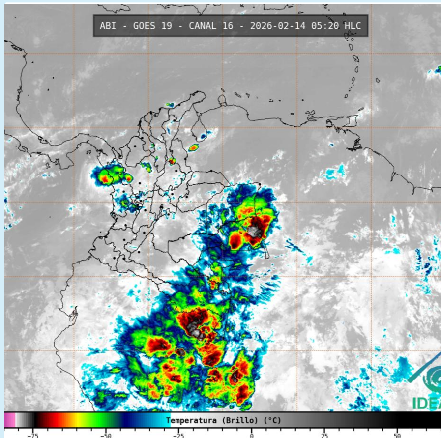
Imagen GOES 19 (East) Canal Infrarrojo 14 de febrero de 2026– Hora 05:20 HLC Fuente: IDEAM - GOES 19
