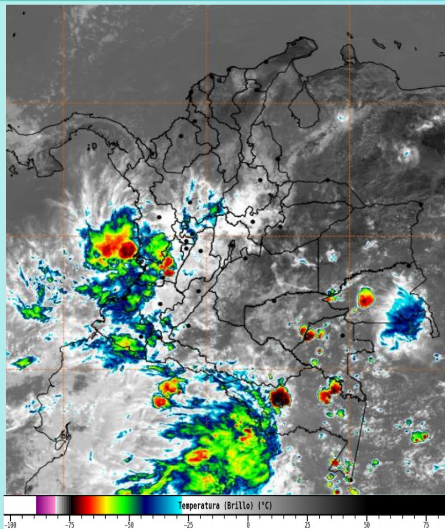
Imagen GOES 19 East Canal Infrarrojo, 13 de febrero de 2026 - Hora 12:00 HLC. Fuente: https://bart.ideam.gov.co GOES 19
