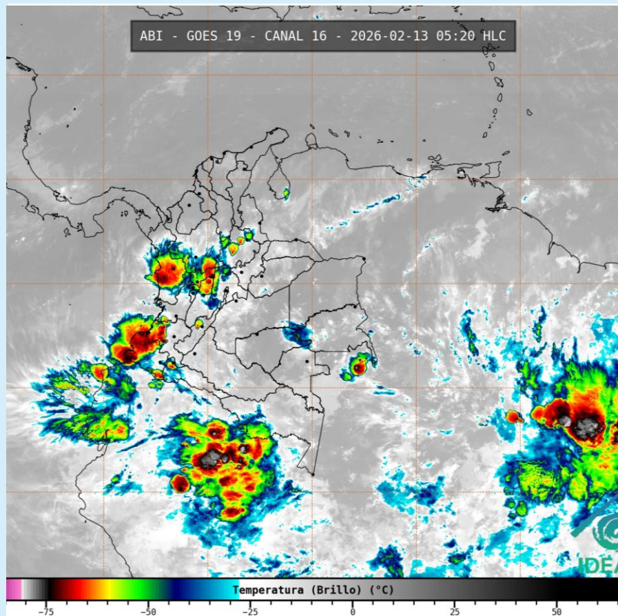
Imagen GOES 19 (East) Canal Infrarrojo 13 de febrero de 2026– Hora 05:20 HLC Fuente: IDEAM - GOES 19
