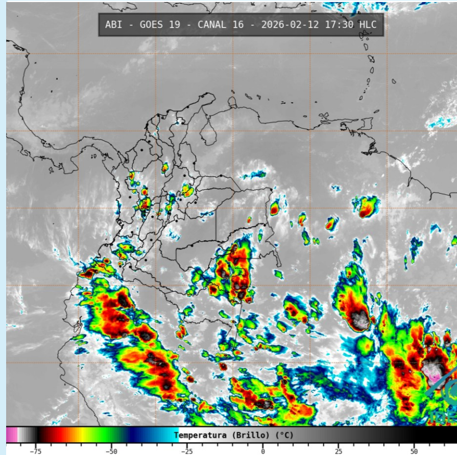
Imagen GOES 19 (East) Canal Infrarrojo 12 de febrero de 2026– Hora 17:30 HLC Fuente: IDEAM - GOES 19
