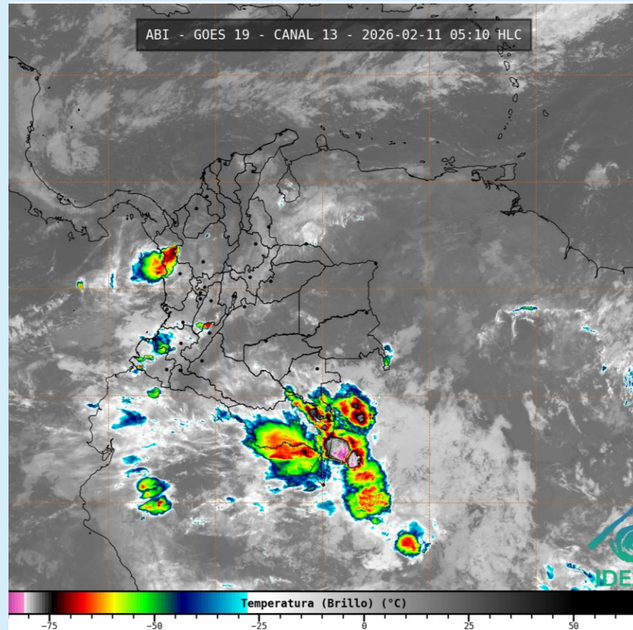
Imagen GOES 19 (East) Canal Infrarrojo 11 de febrero de 2026– Hora 05:10 HLC Fuente: IDEAM - GOES 19
