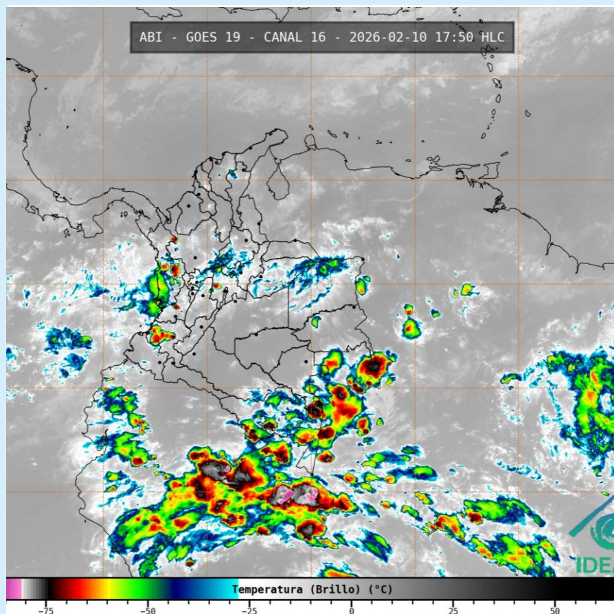
Imagen GOES 19 (East) Canal Infrarrojo 10 de febrero de 2026– Hora 17:50 HLC Fuente: IDEAM - GOES 19
