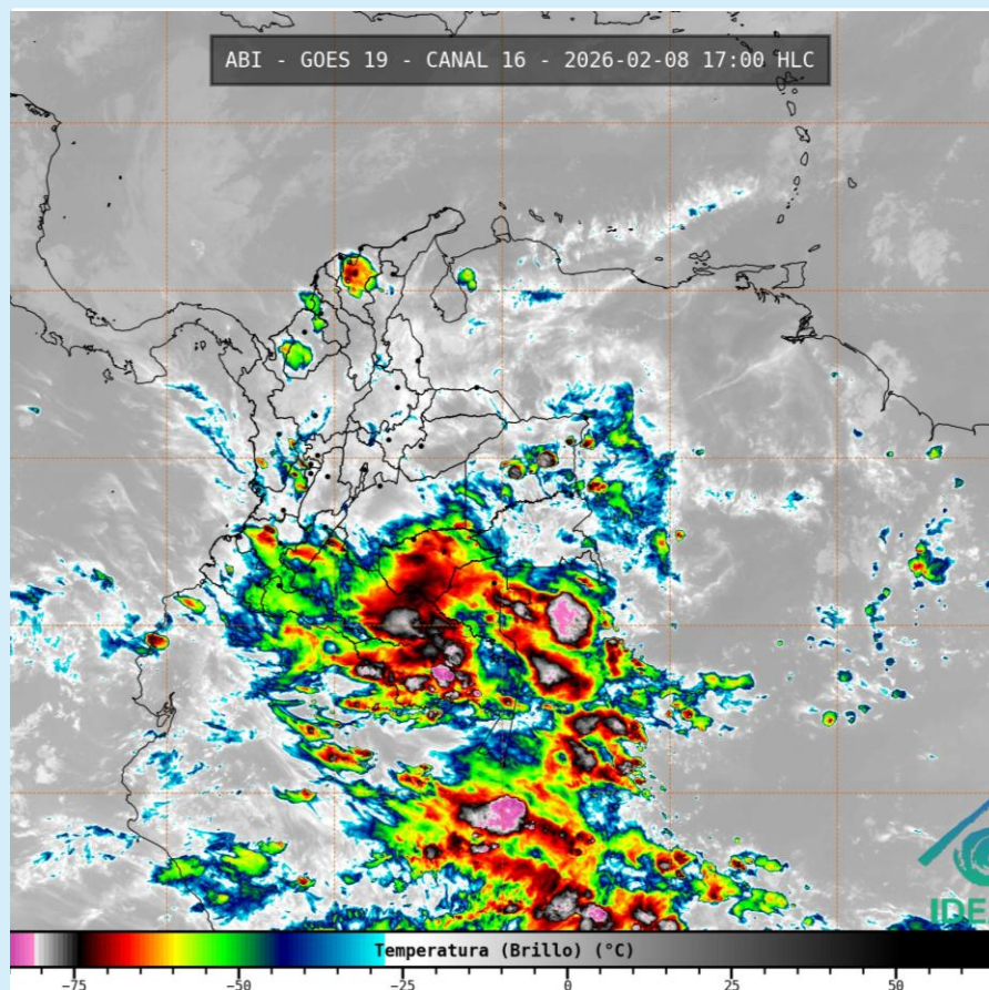
Imagen GOES 19 (East) Canal Infrarrojo 8 de febrero de 2026– Hora 17:00 HLC Fuente: IDEAM - GOES 19
