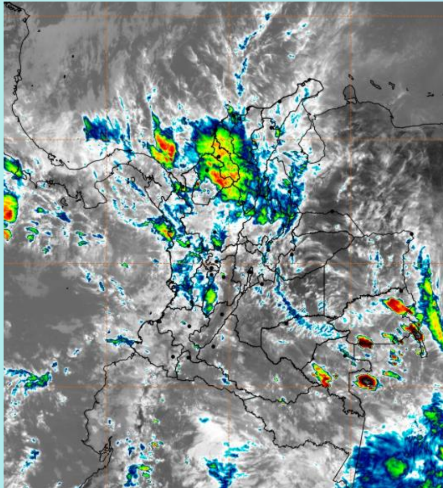
Imagen GOES 19 East Canal Infrarrojo, 6 de febrero de 2026 - Hora 12:40 HLC. Fuente: https://bart.ideam.gov.co GOES 19
