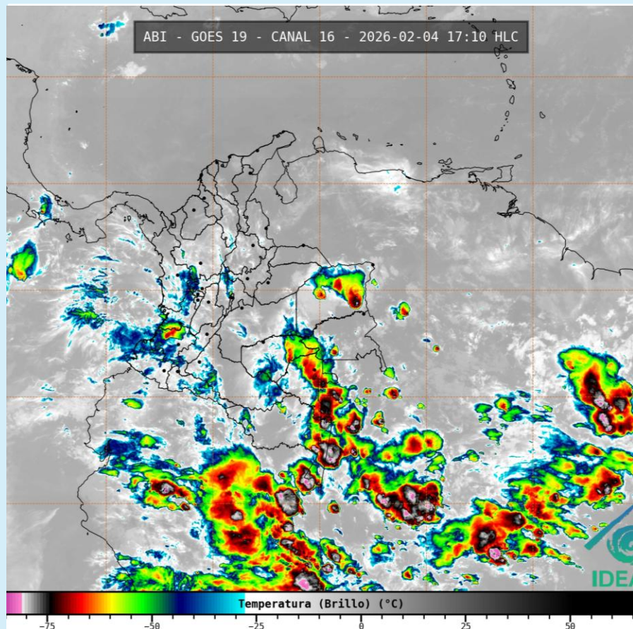
Imagen GOES 19 (East) Canal Infrarrojo 4 de febrero de 2026– Hora 17:10 HLC Fuente: IDEAM - GOES 19
