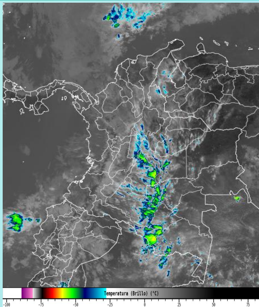
Imagen GOES 19 East Canal Infrarrojo, 3 de febrero de 2026 - Hora 12:00 HLC. Fuente: https://bart.ideam.gov.co GOES 19
