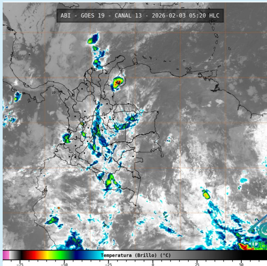
Imagen GOES 19 (East) Canal Infrarrojo 3 de febrero de 2026– Hora 05:20 HLC Fuente: IDEAM - GOES 19
