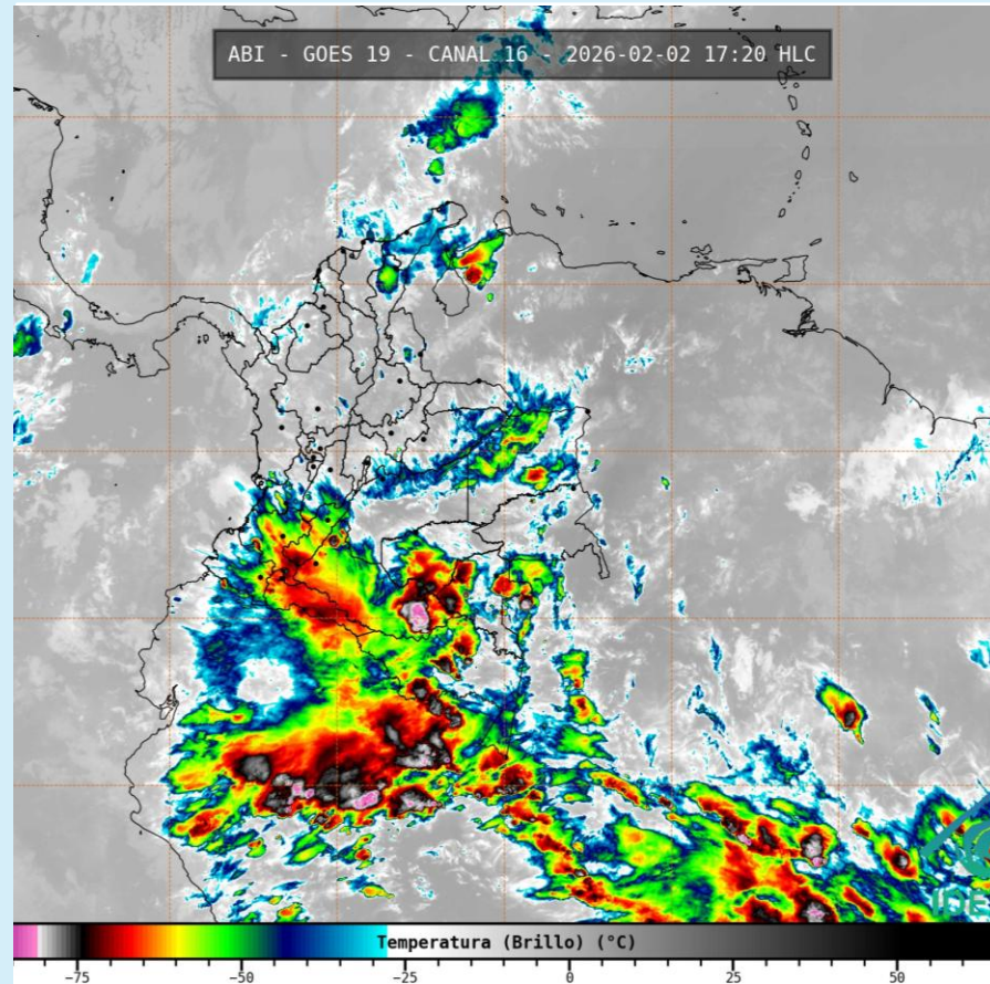
Imagen GOES 19 (East) Canal Infrarrojo 2 de febrero de 2026– Hora 17:20 HLC Fuente: IDEAM - GOES 19
