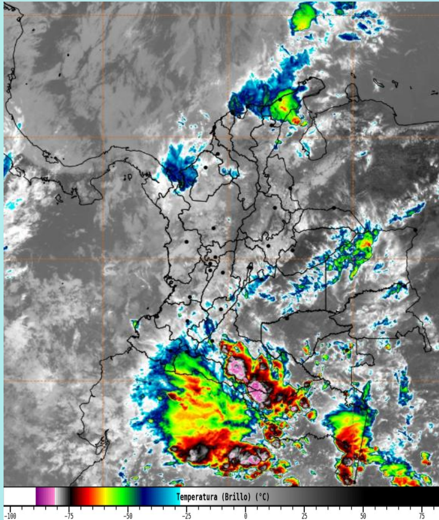
Imagen GOES 19 East Canal Infrarrojo, 2 de febrero de 2026 - Hora 13:20 HLC. Fuente: https://bart.ideam.gov.co GOES 19
