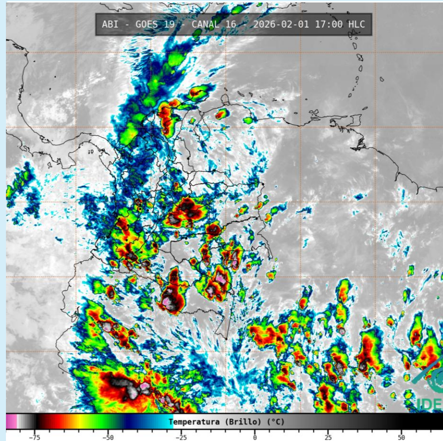
Imagen GOES 19 (East) Canal Infrarrojo 1 de febrero de 2026- Hora 17:00 HLC Fuente: IDEAM - GOES 19
