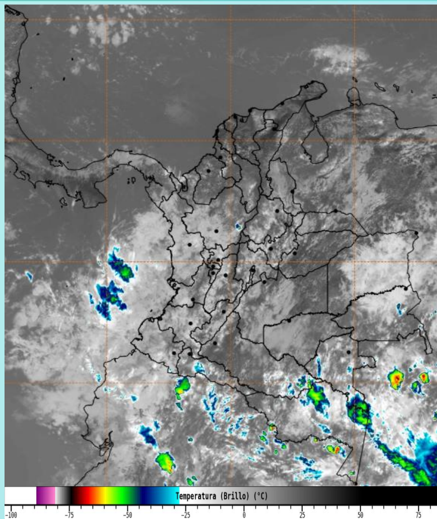
Imagen GOES 19 East Canal Infrarrojo, 26 de enero de 2026 - Hora 12:00 HLC. Fuente: https://bart.ideam.gov.co GOES 19
