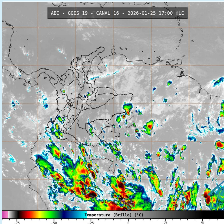
Imagen GOES 19 (East) Canal Infrarrojo 25 de enero de 2026– Hora 17:00 HLC Fuente: IDEAM - GOES 19
