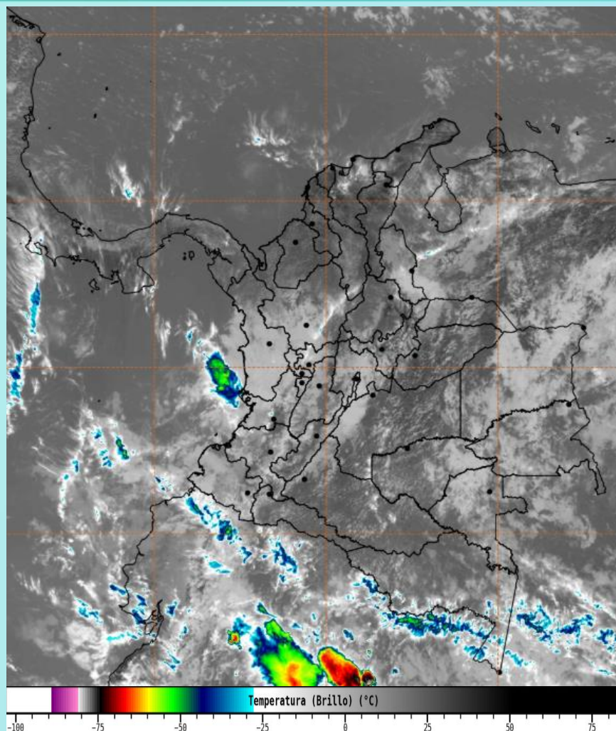
Imagen GOES 19 East Canal Infrarrojo, 25 de enero de 2026 - Hora 12:00 HLC. Fuente: https://bart.ideam.gov.co GOES 19
