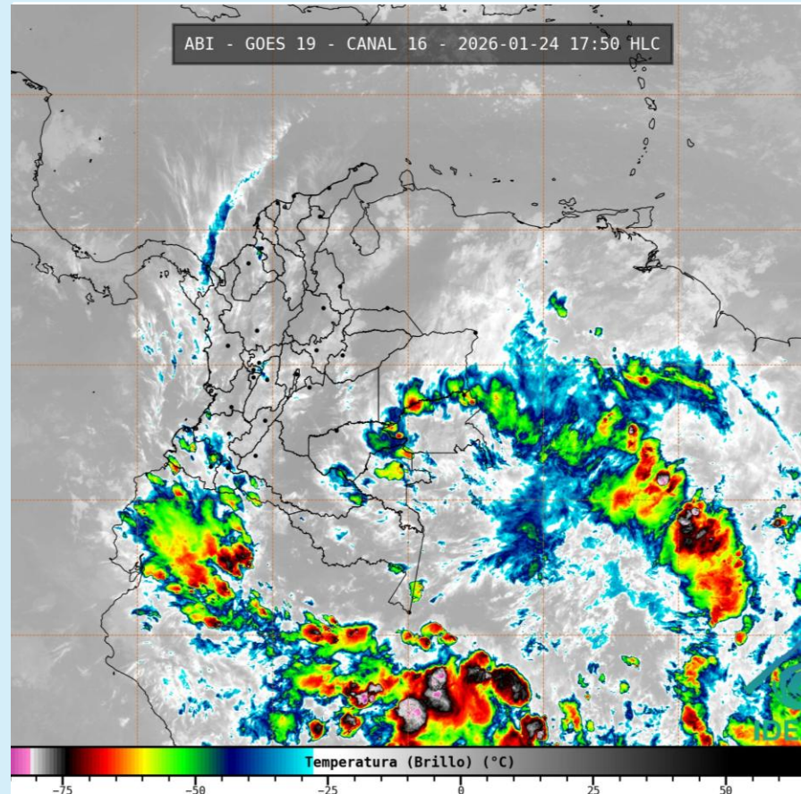
Imagen GOES 19 (East) Canal Infrarrojo 24 de enero de 2026– Hora 17:50 HLC Fuente: IDEAM - GOES 19
