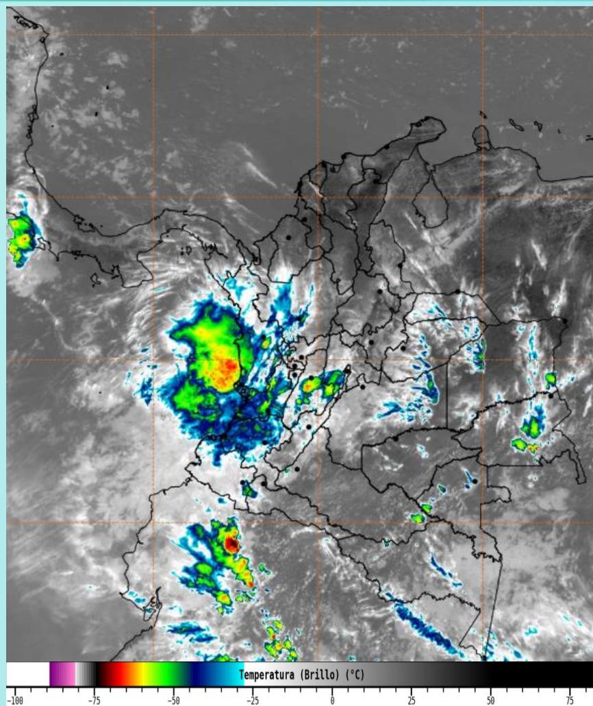
Imagen GOES 19 East Canal Infrarrojo, 22 de enero de 2026 - Hora 12:00 HLC. Fuente: https://bart.ideam.gov.co GOES 19
