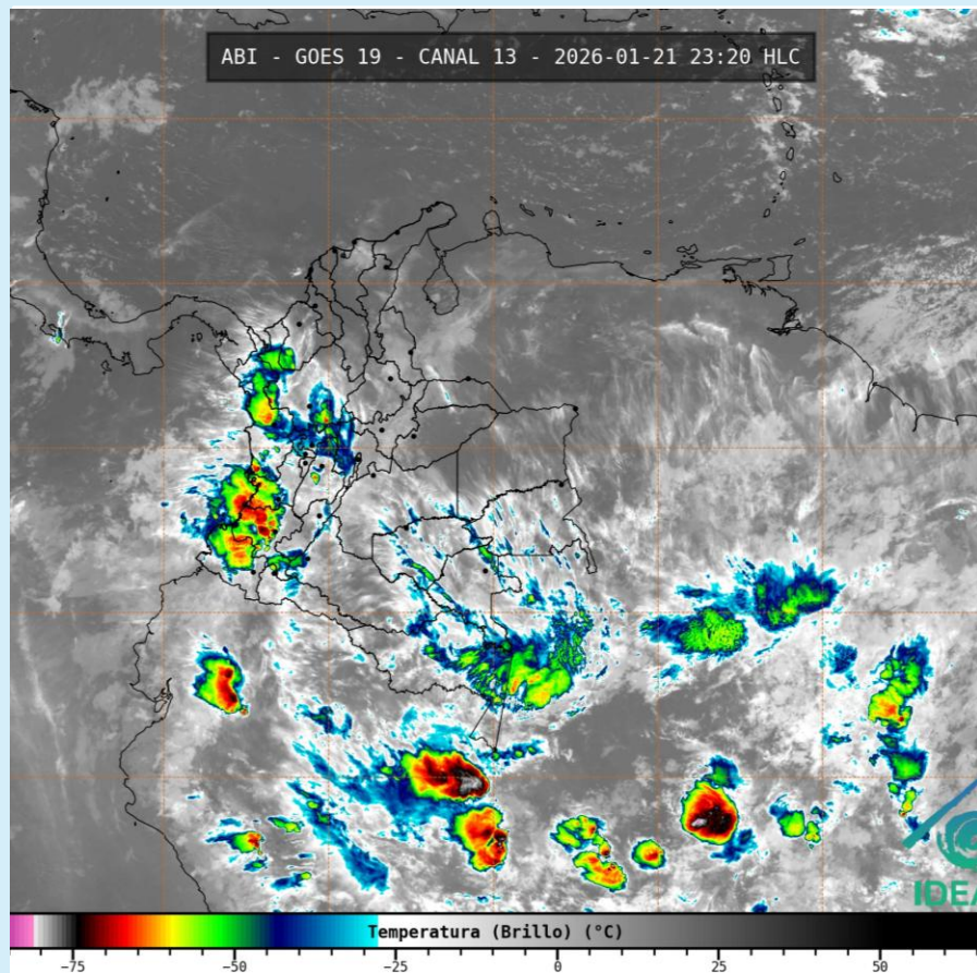
Imagen GOES 19 (East) Canal Infrarrojo 21 de enero de 2026– Hora 23:20 HLC Fuente: IDEAM - GOES 19
