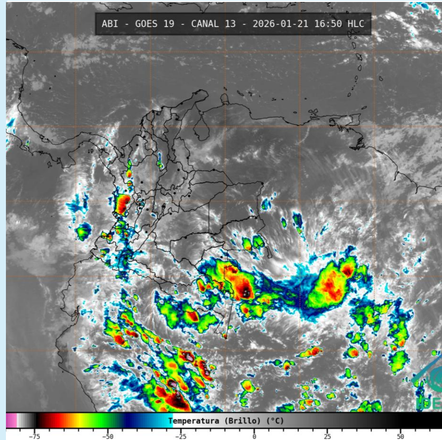
Imagen GOES 19 (East) Canal Infrarrojo 21 de enero de 2026– Hora 16:50 HLC Fuente: IDEAM - GOES 19
