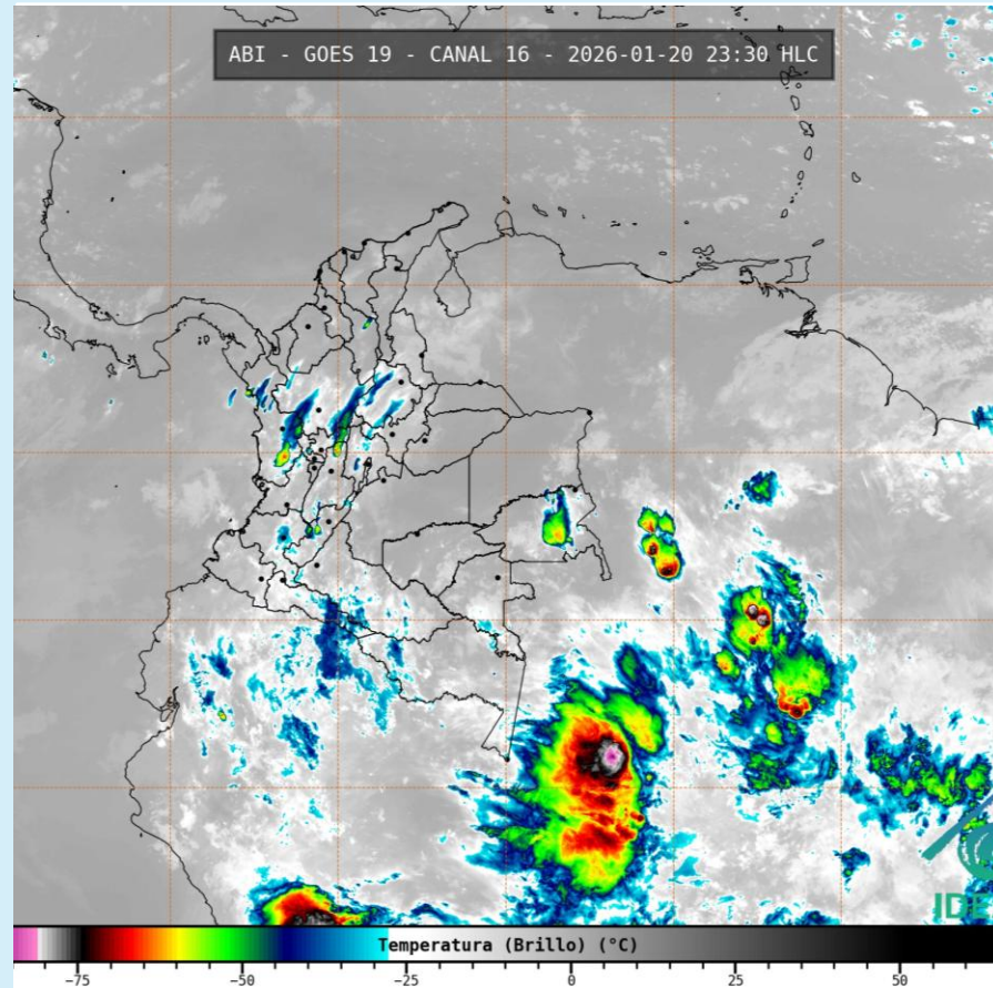
Imagen GOES 19 (East) Canal Infrarrojo 20 de enero de 2026– Hora 23:30 HLC Fuente: IDEAM - GOES 19
