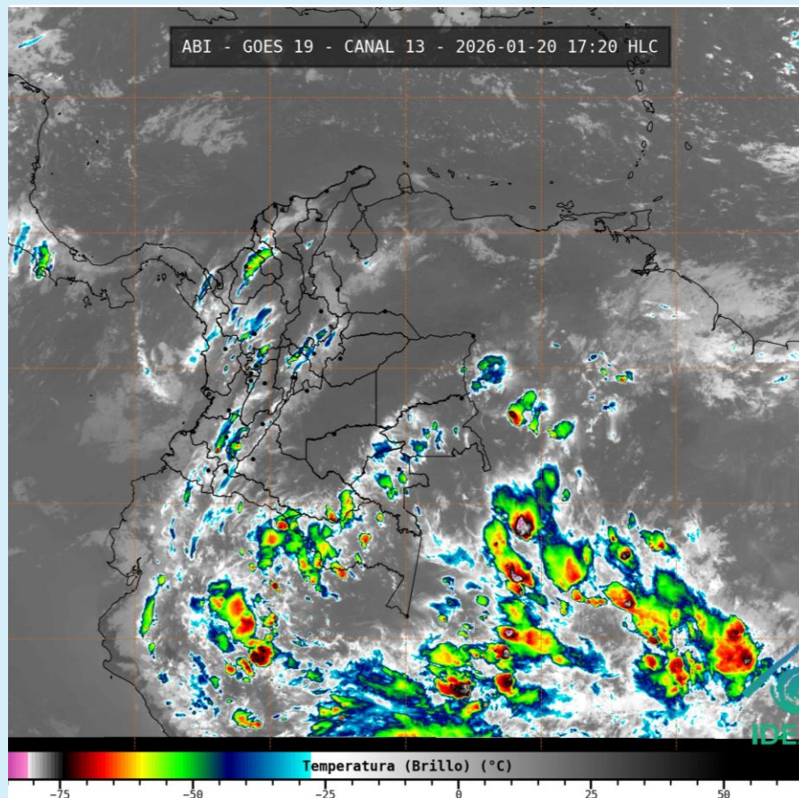
Imagen GOES 19 (East) Canal Infrarrojo 20 de enero de 2026– Hora 17:20 HLC Fuente: IDEAM - GOES 19
