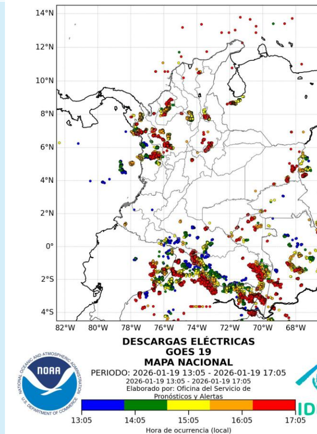
Descargas eléctricas (últimas horas) 19 de enero de 2026 – Hora entre las 13:05 - 17:05 HLC Fuente: IDEAM - NOAA
