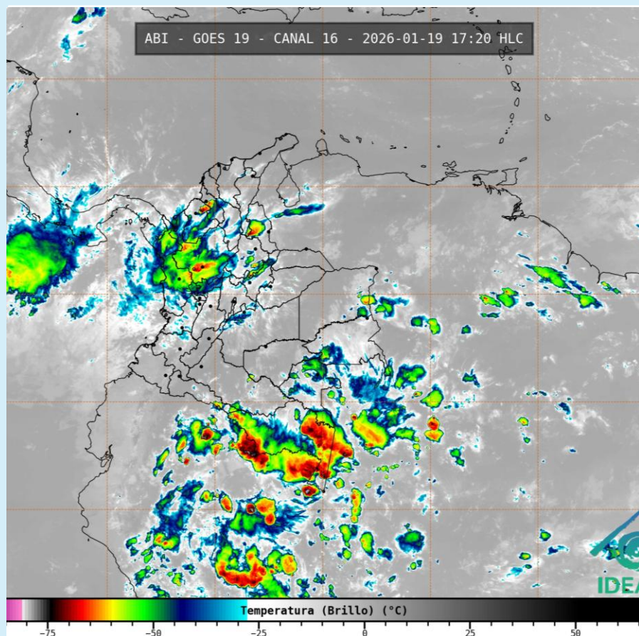
Imagen GOES 19 (East) Canal Infrarrojo 19 de enero de 2026– Hora 17:20 HLC Fuente: IDEAM - GOES 19
