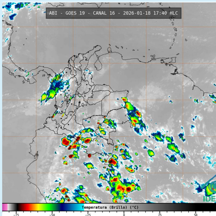
Imagen GOES 19 (East) Canal Infrarrojo 18 de enero de 2026– Hora 17:40 HLC Fuente: IDEAM - GOES 19
