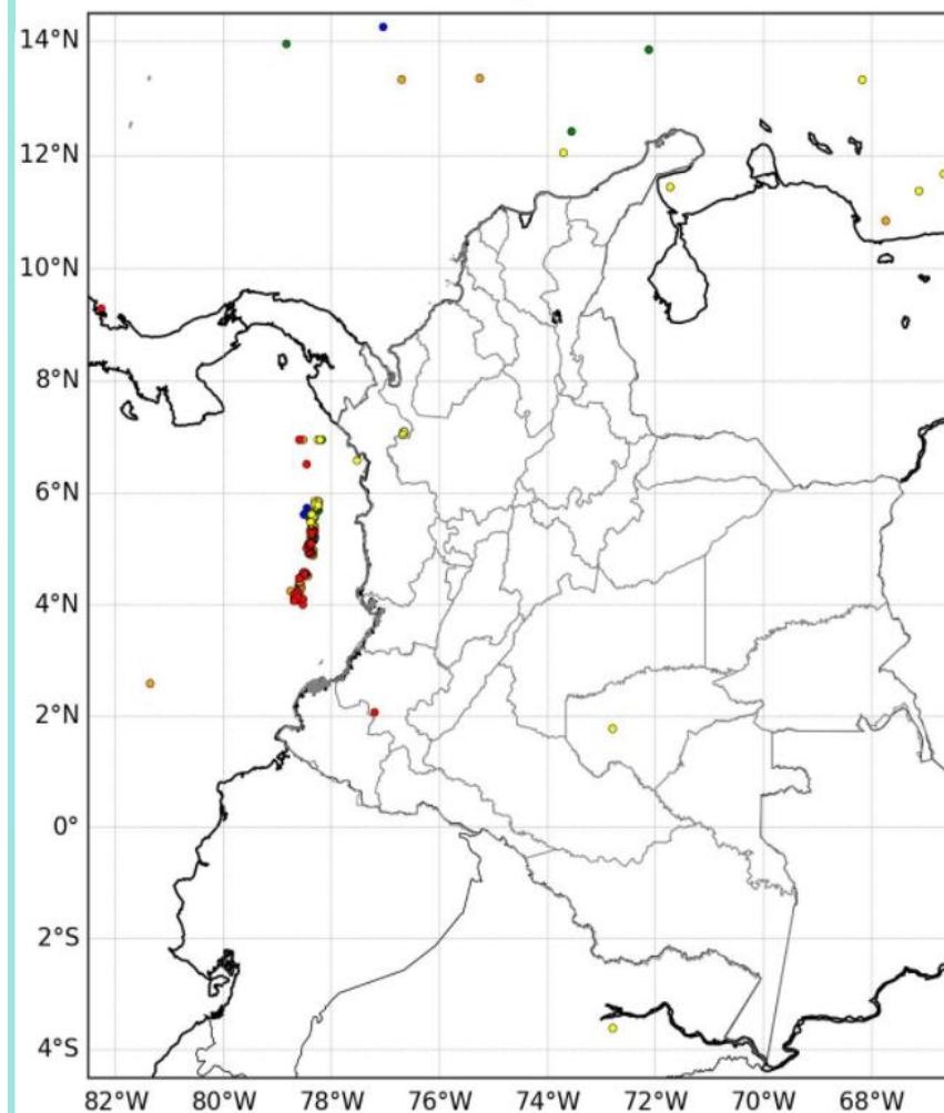
Descargas eléctricas en las últimas 4 horas. Hora 12:00 HLC Fuente: IDEAM - GOES
