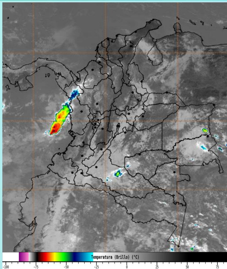
Imagen GOES 19 East Canal Infrarrojo, 18 de enero de 2026 - Hora 12:00 HLC. Fuente: https://bart.ideam.gov.co GOES 19
