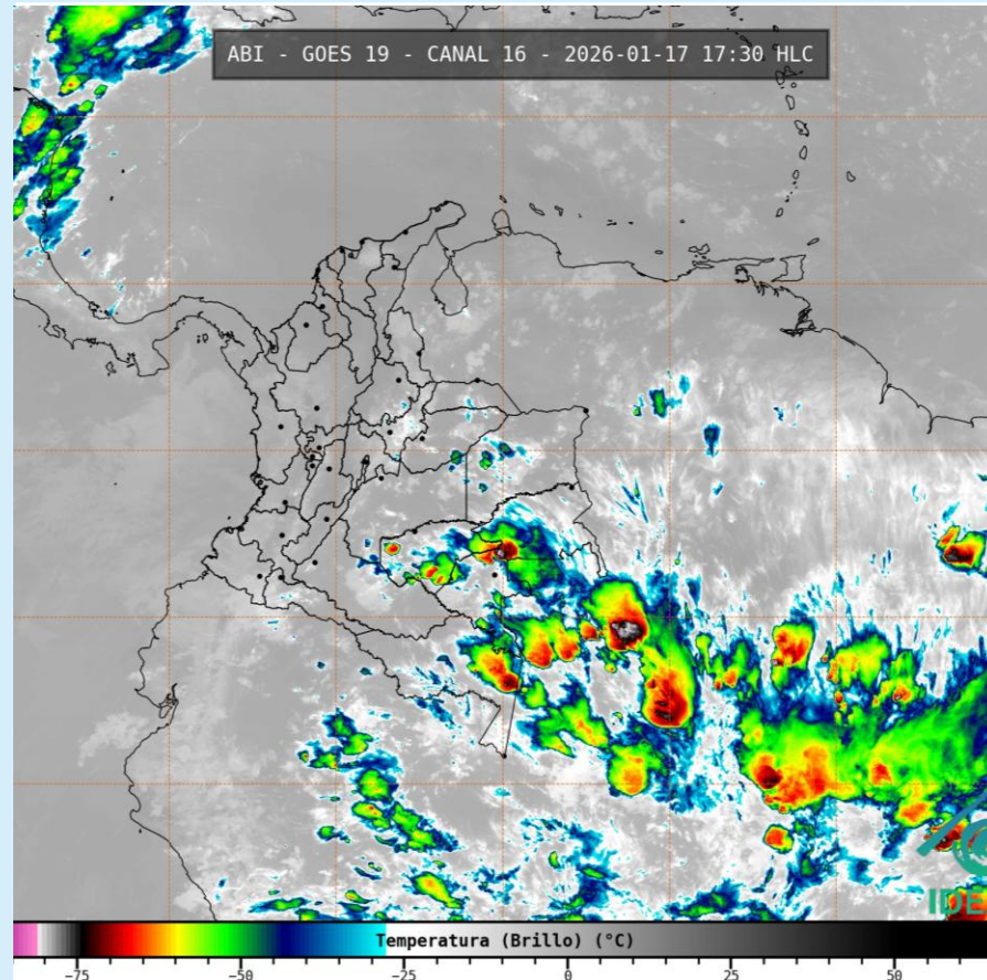
Imagen GOES 19 (East) Canal Infrarrojo 17 de enero de 2026– Hora 17:30 HLC Fuente: IDEAM - GOES 19
